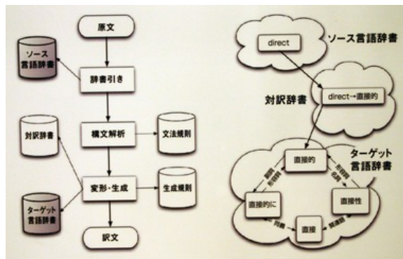
武倉広幸氏が開発した翻訳ソフトのシステム図
